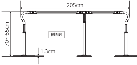
ロング2050タイプ 片手すり XPN-L80605
